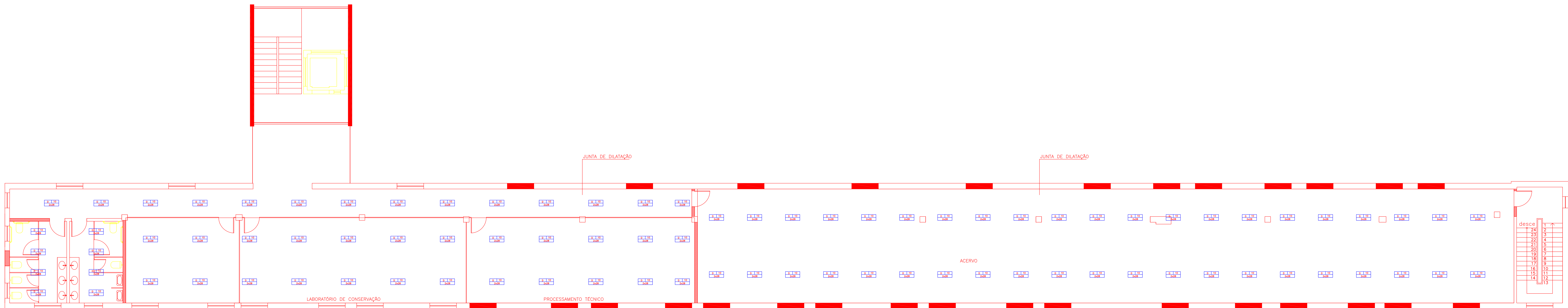
03 PLANTA ANEXO 3 – LUMINOTÉCNICO ESC.: 1/125
