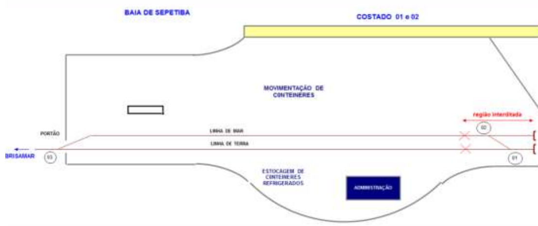
Figura 58 – Vias ferroviárias do píer do Tecon
